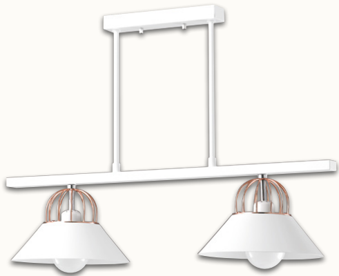
LD 아치(B) 2등 직부(P/D) (백색) ▶Size : W750×D250×H550 ▶Lamp : E26
